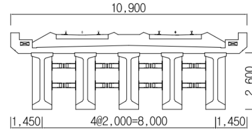
< 강관가로보 >
