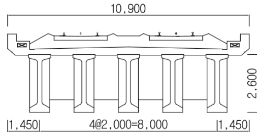
< 콘크리트 격벽 >
