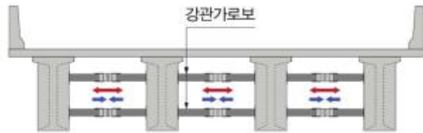
<횡 단 면 도>
