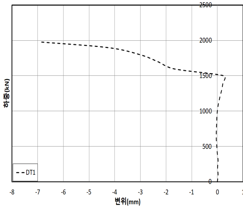
하중-횡변위 곡선
