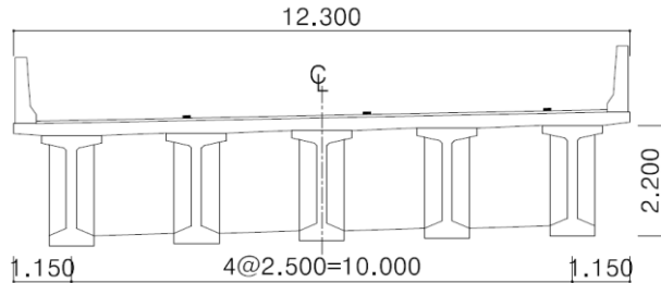
< 콘크리트 격벽 >
