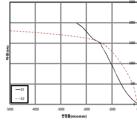
<강관하단부>
