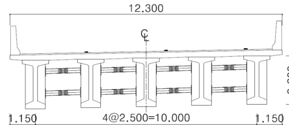
< 강관가로보 >
